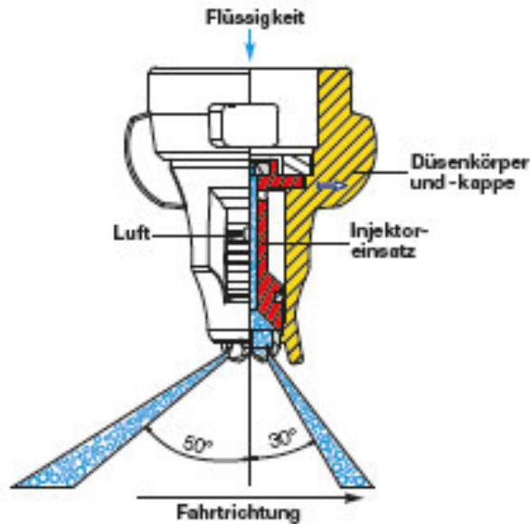
Werkzeuglos herausnehmbarer Injektor
