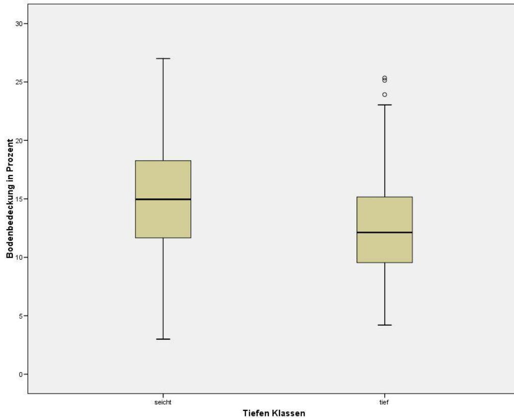
Abbildung 35: Einfluss der Bearbeitungstiefe auf die Bodenbedeckung
